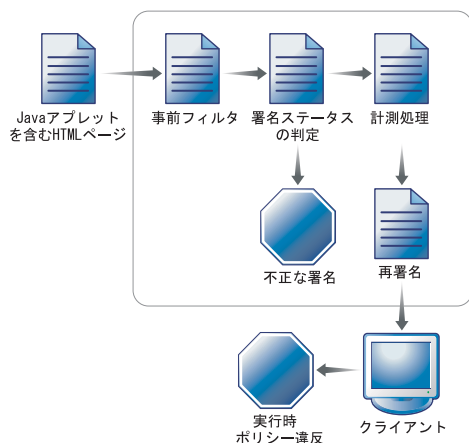
図 4-3. Java アプレット対策の仕組み
