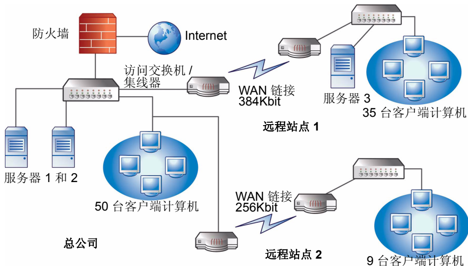
图 A-2 多个站点网络拓扑
